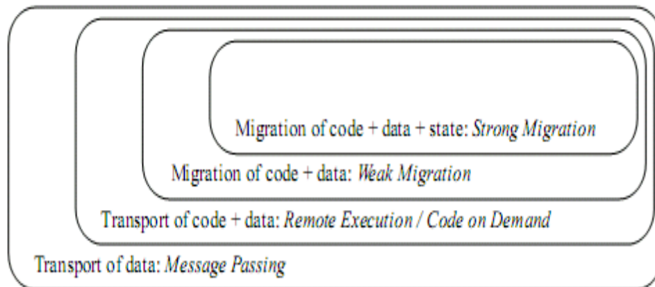
Gambar 2. Tingkatan pergerakan (Kurt Rothermel and Markus Schwehm, 1998)
