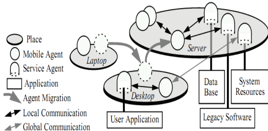
Gambar 3: Sistem agen bergerak (Kurt Roethermel and Markus Schwehm, 1998)
