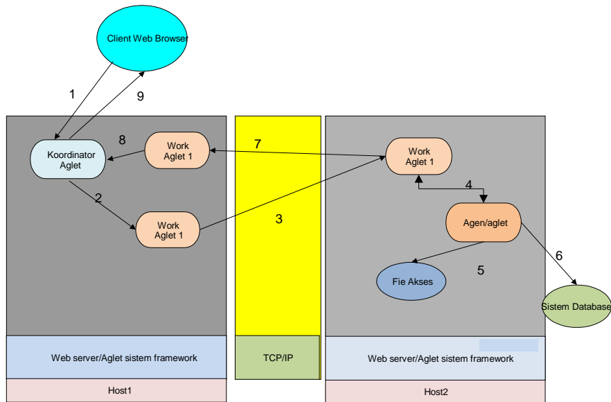
Gambar 8: konsep proses pencarian file dengan Aglet
